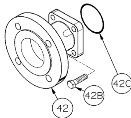
ANSI FLANGE
